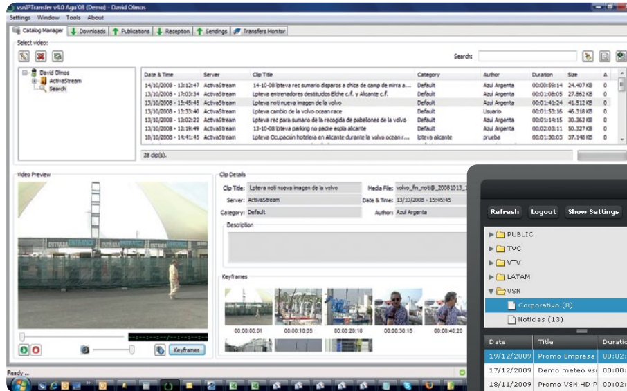
VSNIPTRANSFER interface
