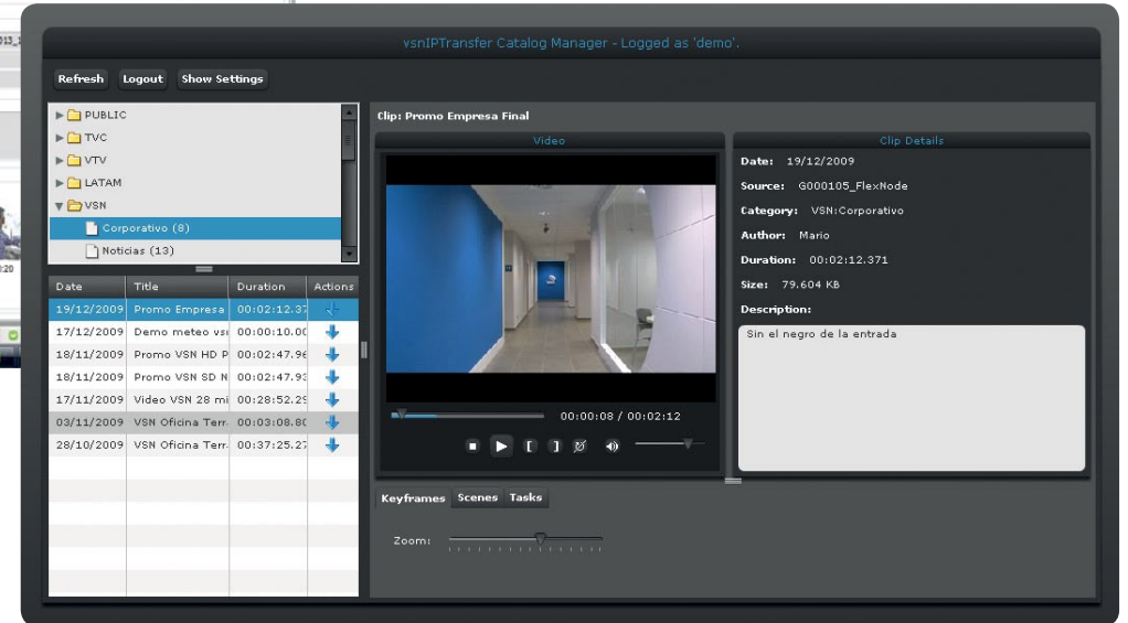
VSNIPTRANSFER interface
