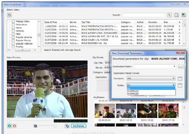
VSNIPTRANSFER interface
